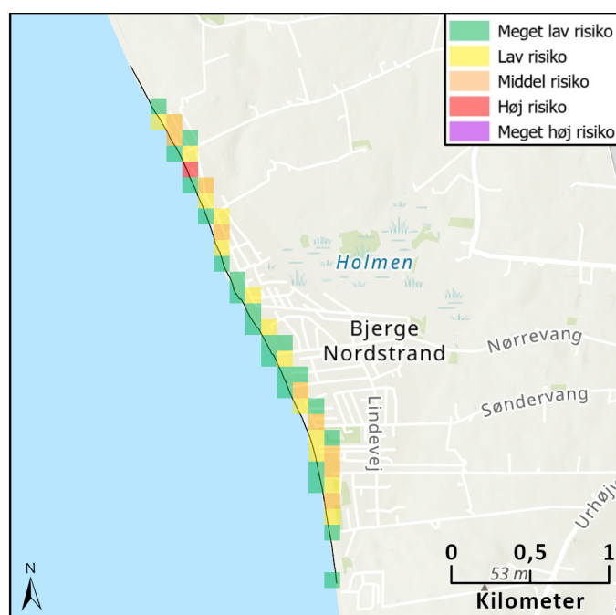
Figur 7 Risikokort, erosion
