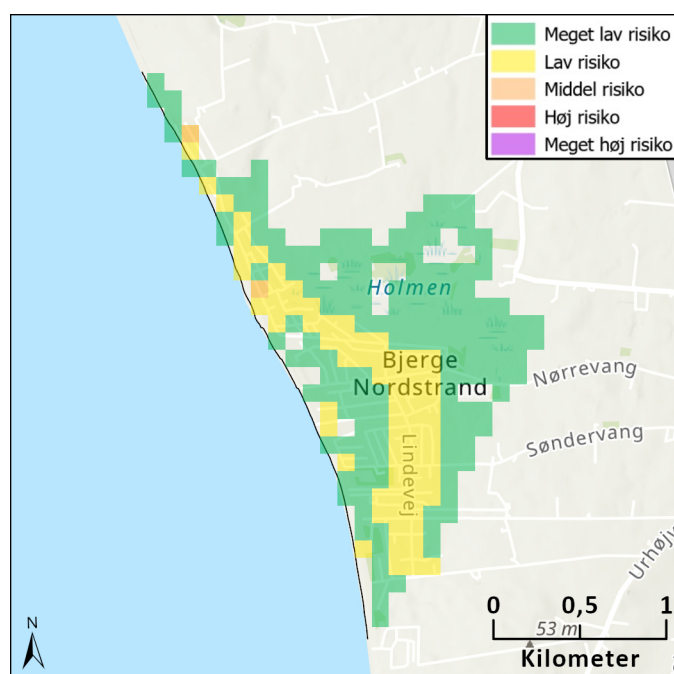
Figur 6 Risikokort, oversvømmelse
