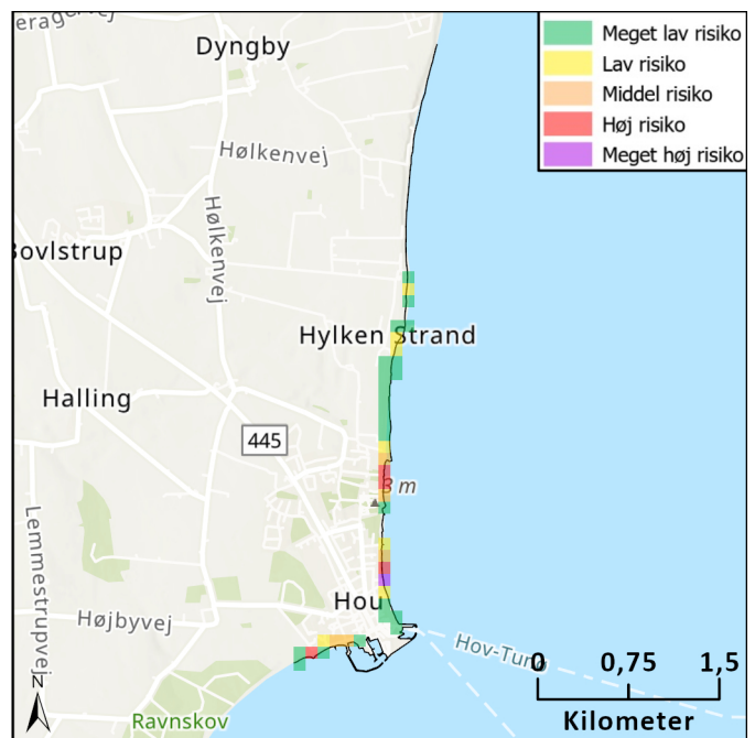
Figur 5 Risikokort, erosion
