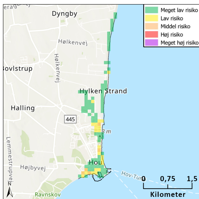
Figur 2 Risikokort, oversvømmelse
