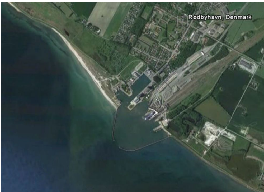
Figur 4.15 Luvside tilsanding nordvest for Rødbyhavn, hvor der er en netto langstransport på ca. 30.000 m 3 /år imod sydøst fremkaldt af fremherskende bølger fra vestlige retninger. Området sydøst for havnen er omvendt under erosion.
