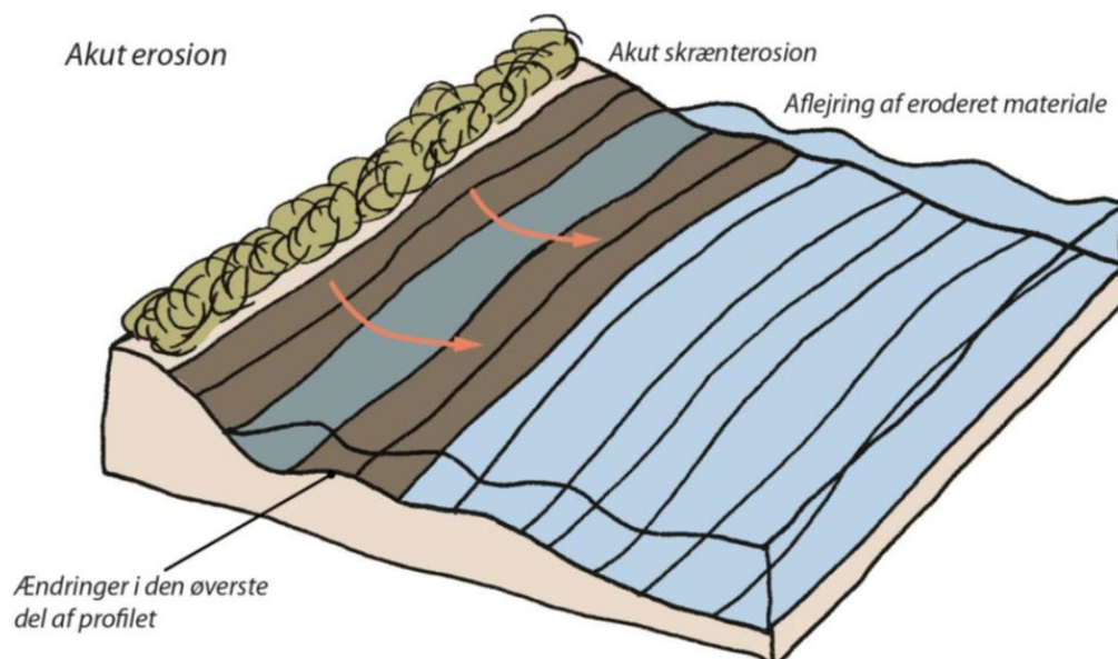
Figur 4.16 Under akut erosion eroderes den øvre del af profilet ved højvande (storm). Det eroderede materiale lægger sig ud i de dybere dele af kystprofilet. Mørk brun og mørkeblå viser, hvor profilet er aktivt under akut erosion. Det lyseblå område er ikke aktivt.
