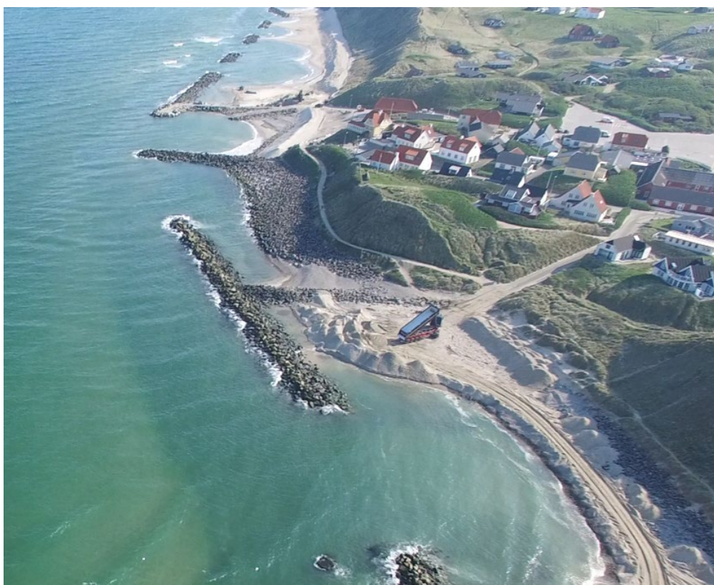
Figur 5.4 Bølgebryder hvor erosionen forøges, fordi kystens orientering ændres. Der kompenseres for erosionen med sandfodring som det ses midt i billedet.
